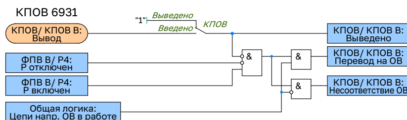
Рисунок 2.66 – Функциональная схема логики контроля перевода на ОВ
