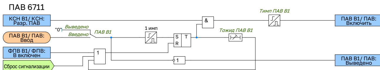
Рисунок 2.50 – Функциональная схема логики ПАВ
