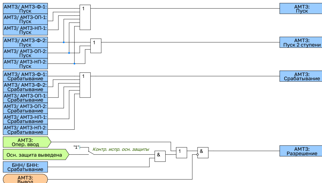
Рисунок 2.31 – Функциональная схема общей логики АМТЗ
